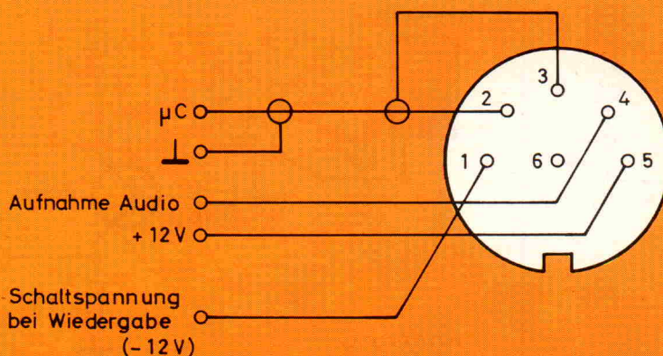
Bild 4. Belegung einer DIN-VCR- Buchse. Der von uns mit \mu\text{C} bezeichnete Pin wird mit dem Videoausgang des Rechners verbunden.
