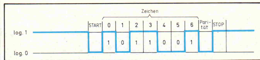
Bild 3. Leitungspegel beim Senden des Zeichens 'M' (hexa 4D, gerade Parität, 1 STOP-Bit)
