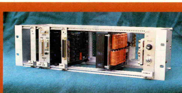
Bild 6. Die Mikro-Busplatine ermöglicht die Verwendung von Flachsteckverbindungen. Bei Kontaktschwierigkeiten sollten die Stecker auf der anderen Seite der Platine montiert werden.
