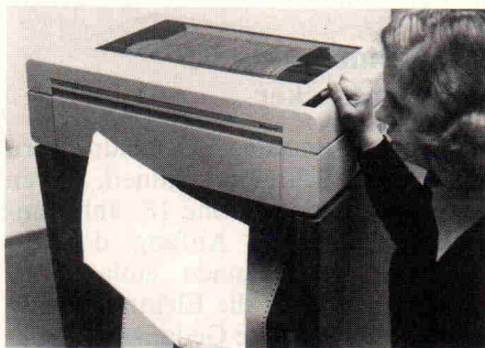
Matrixdrucker mit 9x7-Matrix (Foto: Siemens)
